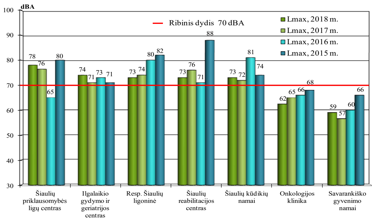
108 pav. Maksimalaus triukšmo lygis kitimas ligoninių, gydymo įstaigų aplinkoje 2015÷2018 m.
