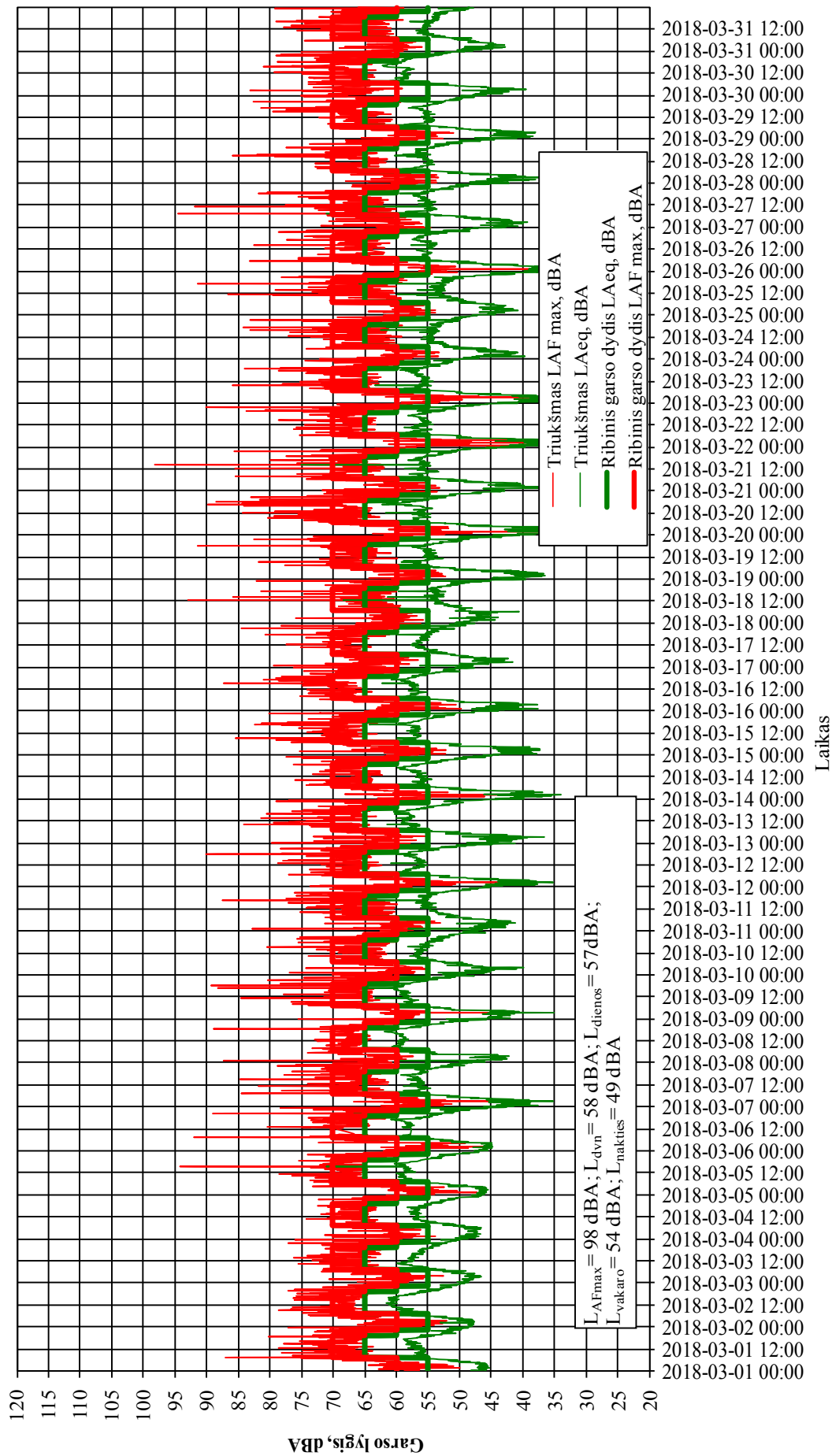
121 pav. Nuolatinių triukšmo matavimų duomenys pietiniame gyvenamajame rajone (Gegužių g. 94) 2018 m. kovo mėn.
