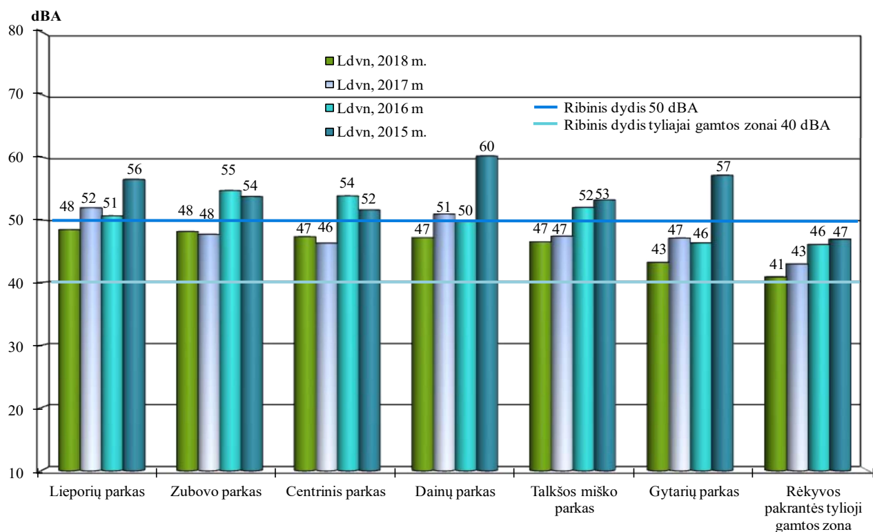
111 pav. Ekvivalentinio triukšmo lygio kitimas Šiauliu m. tyliosiose zonose 2015 ÷ 2018 m.
