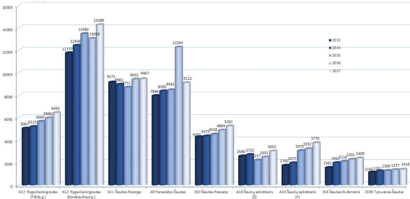
57 pav. Bendrojo vidutinio metinio paros eismo intensyvumo kitimas valstybinės reikšmės keliuose Šiaulių miesto prieigose 2013-2017 m.
